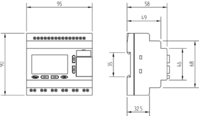
Чертеж 2
