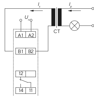
б) с трансформатором тока
