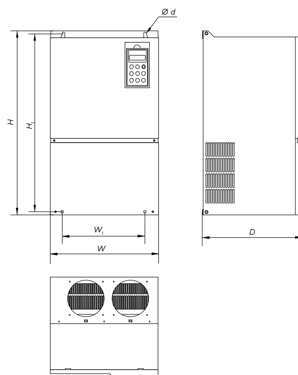
Габарит 5.3
