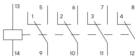
РЭК77/4, РЭК78/4
