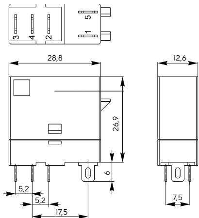
а) Реле общего назначения OGR-11C
