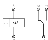
а) подключение к сети постоянного тока
