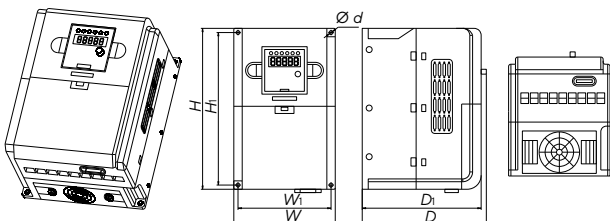
Габарит 3
