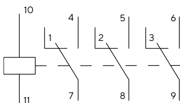
РЭК77/3, РЭК78/3
