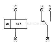
б) подключение к сети переменного тока
