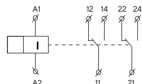
CTR-450-AM-2-20A-U240-C00
