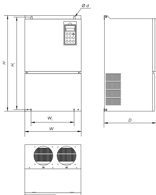
Габарит 5.2
