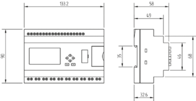
Чертеж 3
