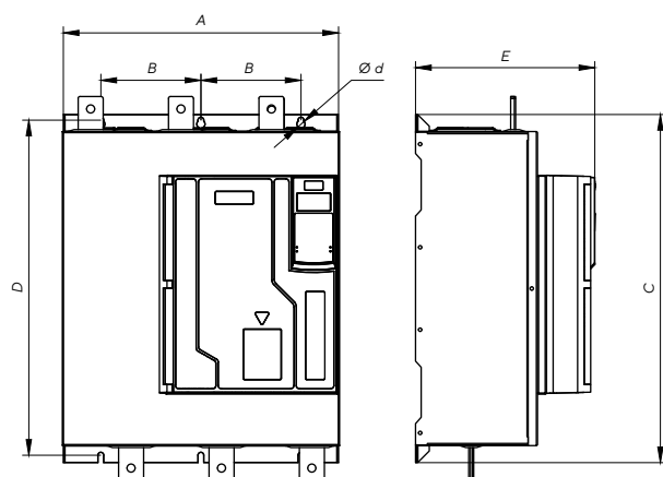
Габарит 3
